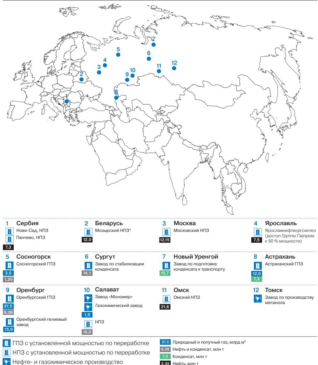
Мощности Группы Газпром по переработке углеводородного сырья, газо- и нефтехимии на 31.12.2014 г.
