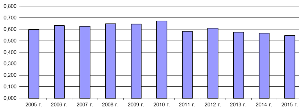
Потребление теплоты на 1 тонну товарной продукции, Гкал/тонна
