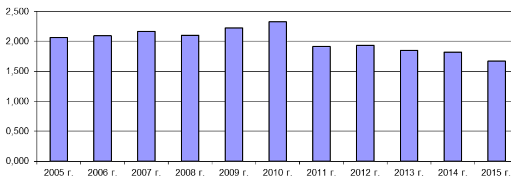
Потребление теплоты на 1 тонну товарной продукции, Гкал/тонна
